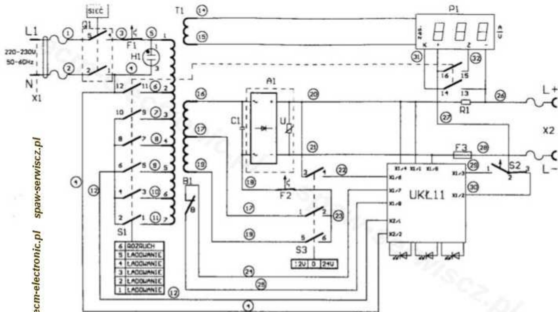
Schemat ideowy zespołu prostownikowego HERKULES 300
